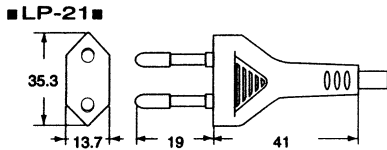
LP-21 (CEE 7 Plug)
